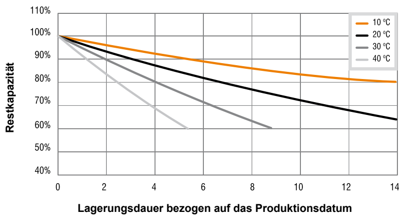
Selbstentladecharakteristik
